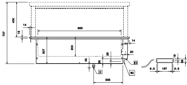
Front aanzicht
