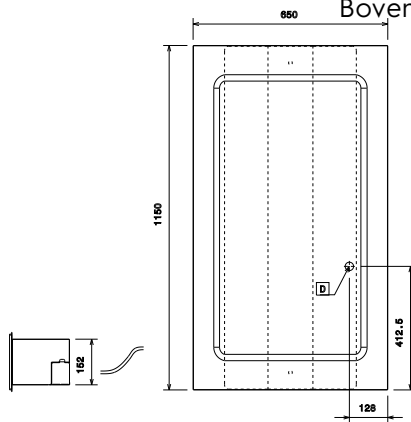
Boven aanzicht
